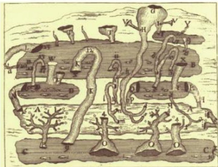
Valvasor si je delovanje Cerkniškega jezera predstavljal kot pet sifoni povezanih podzemnih jezer.
